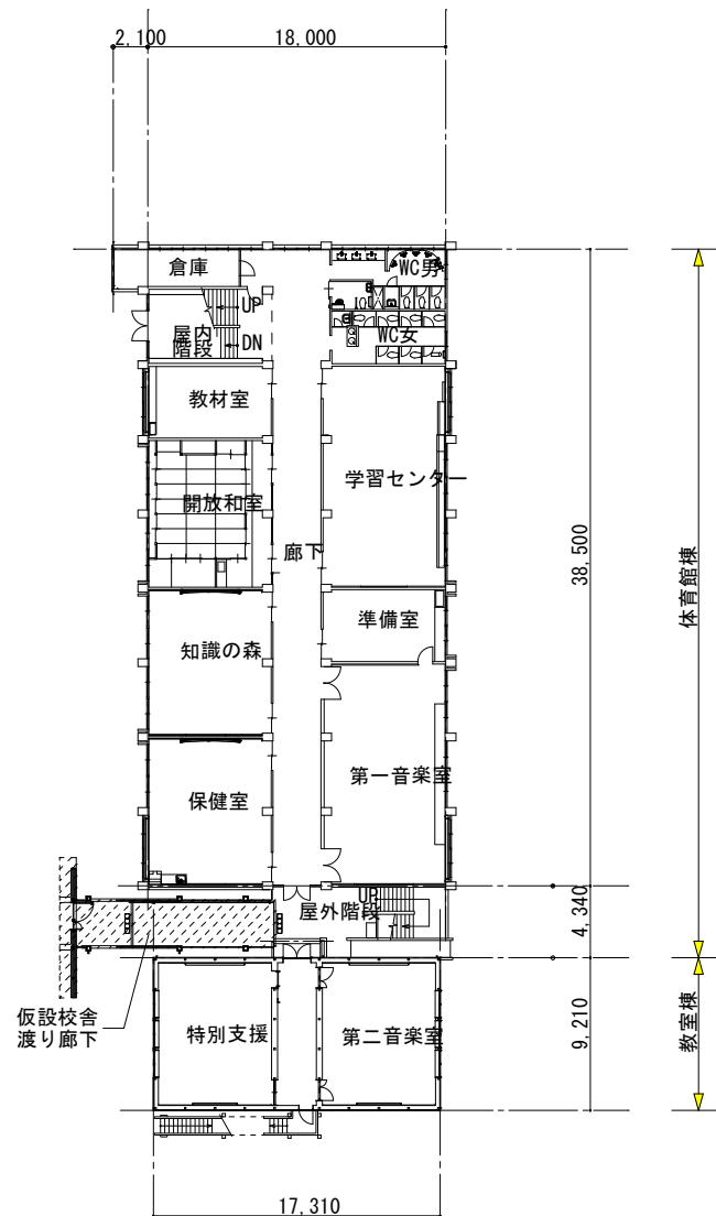
1 階平面図
