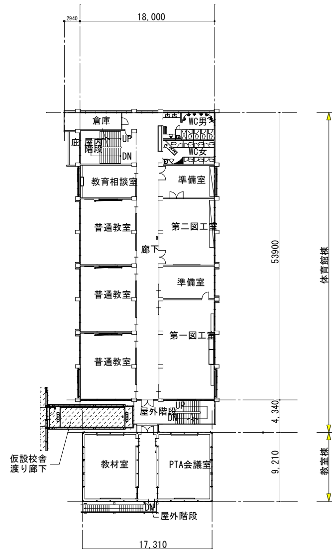
2 階平面図
