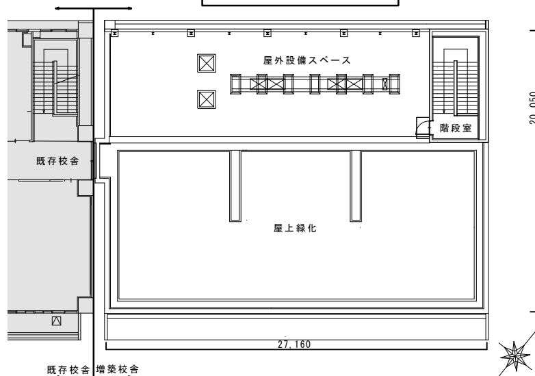
屋上平面図
