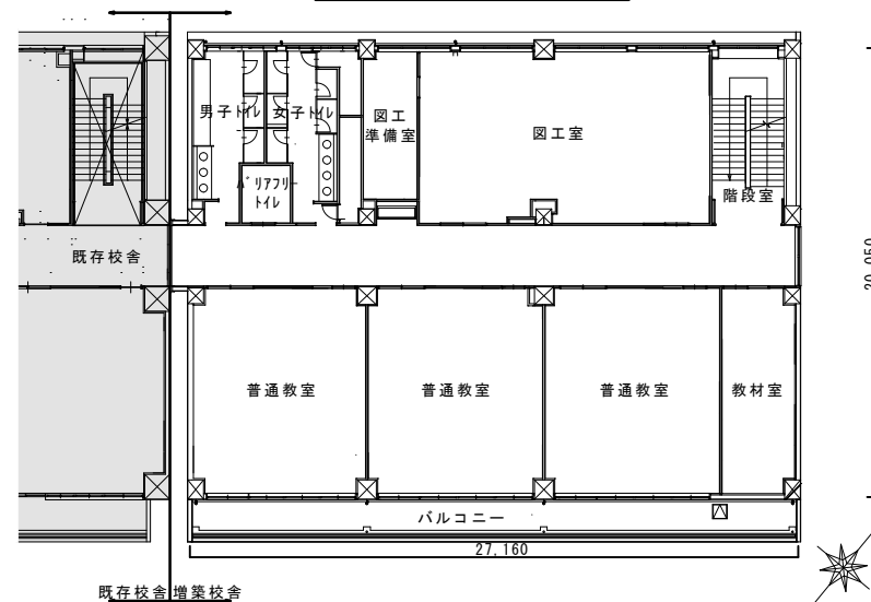
2 階平面図
