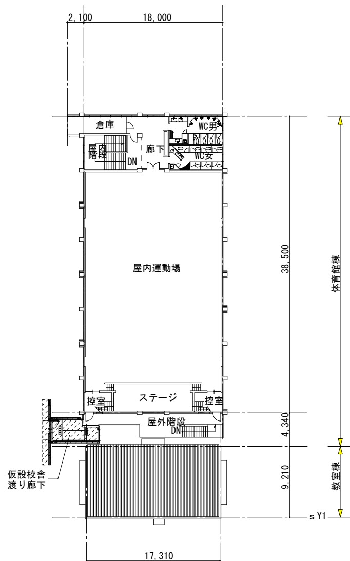
3 階平面図
