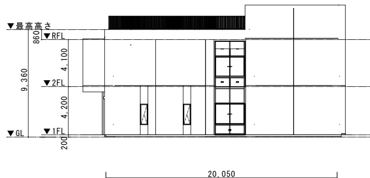
西側立面図
