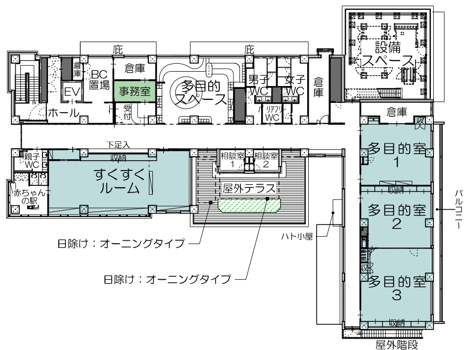
3F 平面
